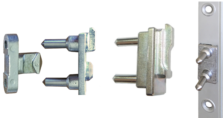
Plantilla clipada, señalizadora de agujeros para los cerraderos del marco
