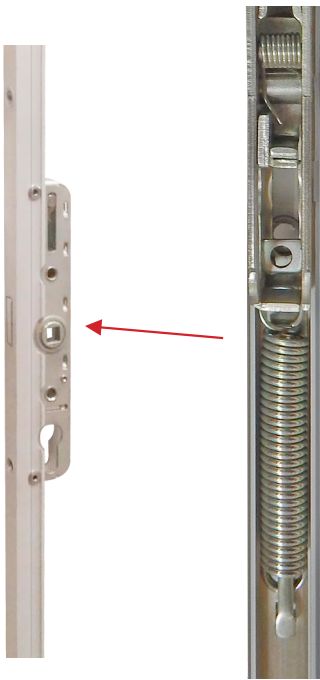
Muelle de retención para recuperación lenta del movimiento de la manilla
